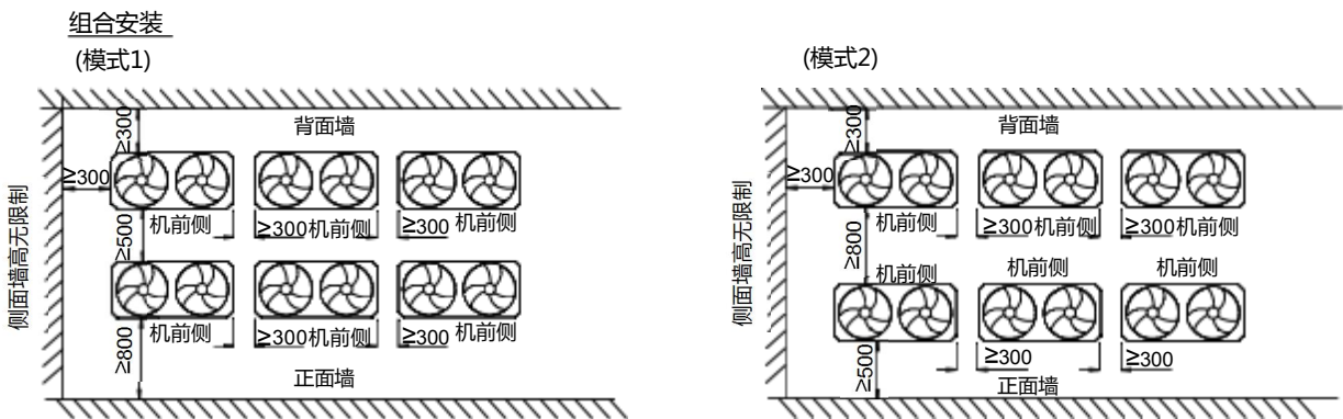
YMAE机组安装空间示意图
