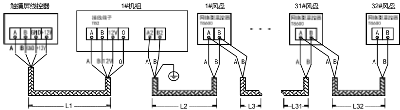
通讯方式风盘联控通讯线连接图
