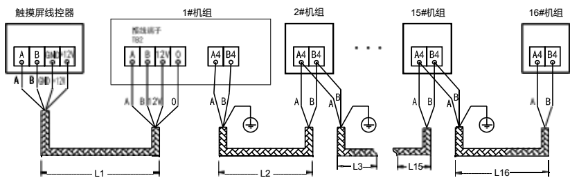
通讯方式风盘联控通讯线连接图
